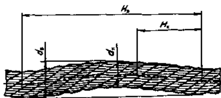
Рис. 2. Волнистость каната
