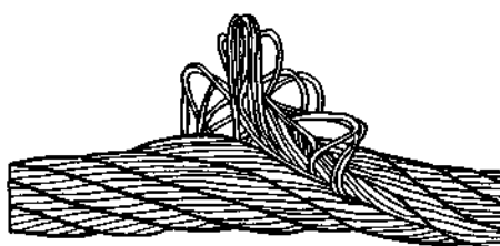
Рис. 4. Выдавливание сердечника
