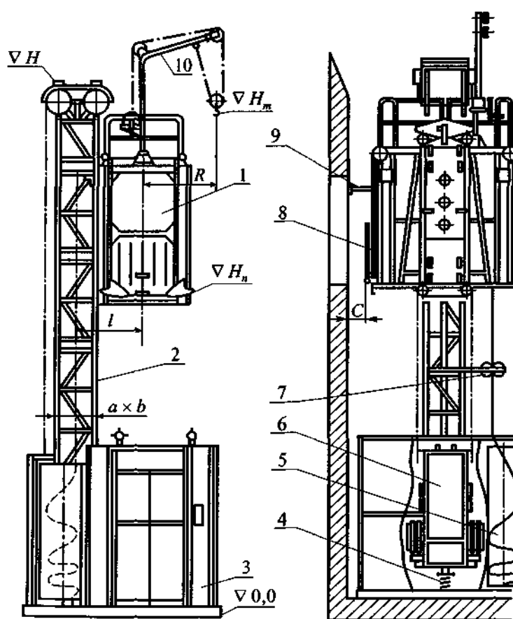
1 — кабина; 2 — мачта; 3 — опорный блок; 4 — буфер; 5 — контейнер электрокабеля; 6 — противовес; 7 — ловушка; 8 — трап; 9 — узел крепления; 10 — устройство монтажное
